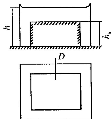
Рис. 3.5. Зона защиты замкнутого тросового молниеотвода
