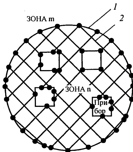
Рис. 4.5. Сетчатое выполнение системы уравнивания потенциалов
