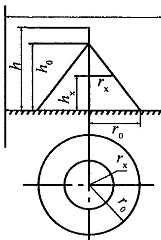
Рис. 3.1. Зона защиты одиночного стержневого молниеотвода
