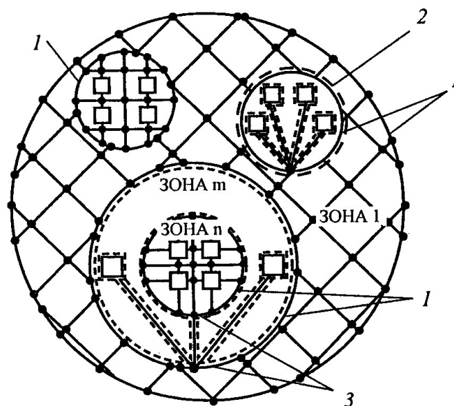
Рис. 4.6. Комплексное выполнение системы уравнивания потенциалов
