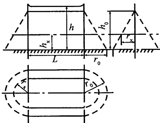
Рис. 3.2. Зона защиты одиночного тросового молниеотвода
