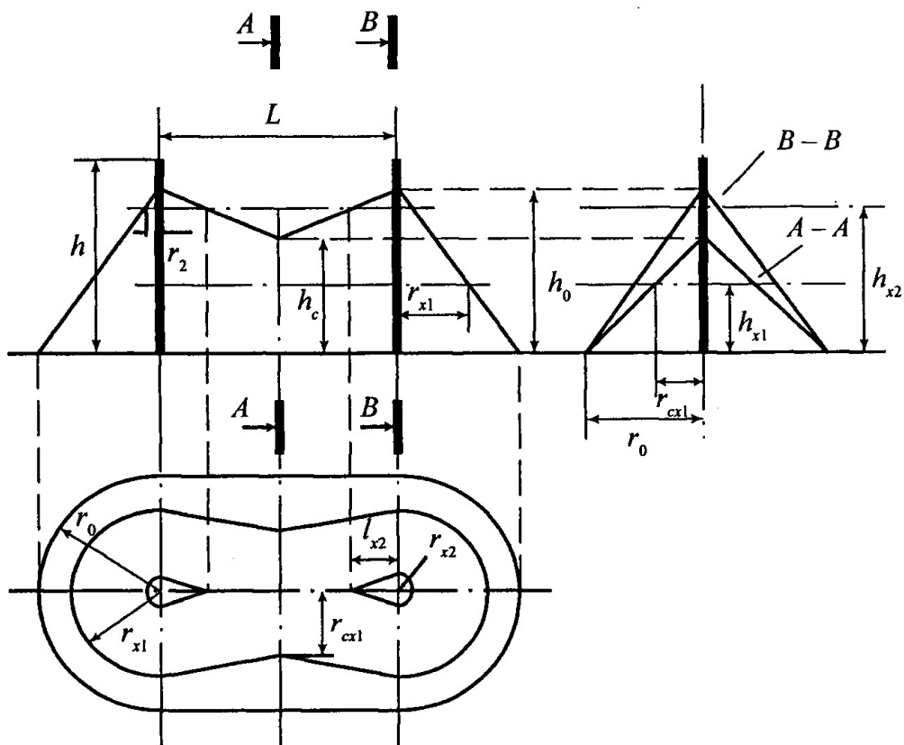
Рис. 3.3. Зона защиты двойного стержневого молниеотвода
