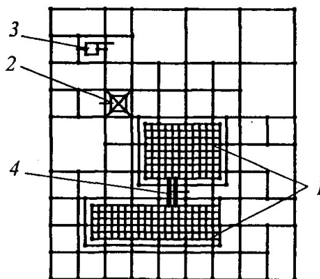
Рис. 4.8. Сетчатое заземляющее устройство производственных сооружений
