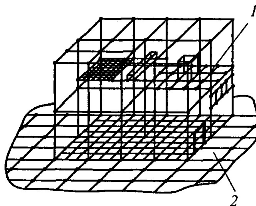
Рис. 4.7. Сетчатое заземляющее устройство здания
