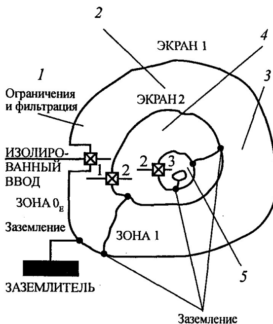
Рис. 4.1. Зоны защиты от воздействия молнии
