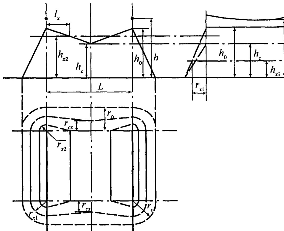
Рис. 3.4. Зона защиты двойного тросового молниеотвода
